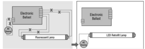
FIG 2 - Retrofit avec 1 lampe
