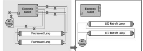
FIG 3 - Reequipamiento con 2 lámparas
